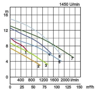
Vortex-juoksupyörä, jossa leveä pumppukotelo, 4-napainen moottori, tukkeutumaton.
