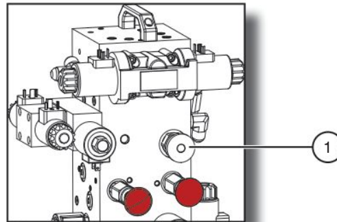
Kuva 2-8. Rullausventtiili
