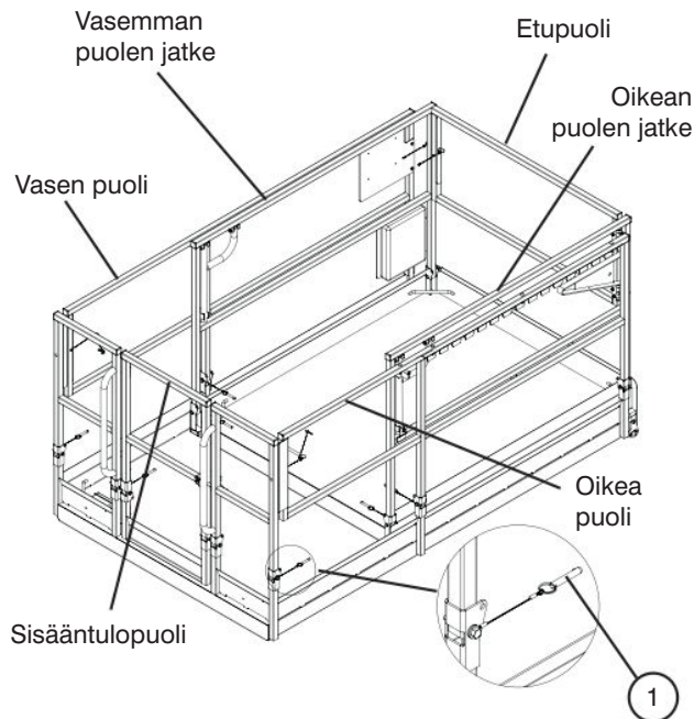
Kuva 3-9a. Taitettavat suojakaiteet
