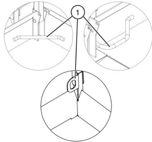
Kuva 3-3. Putoamisenestosuojan kiinnityspiste
