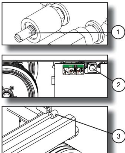
Kuva 2-10. Hätälaskujärjestelmä
