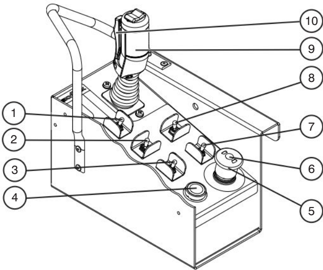
Kuva 2-6. Lavan ohjauspaneeli
