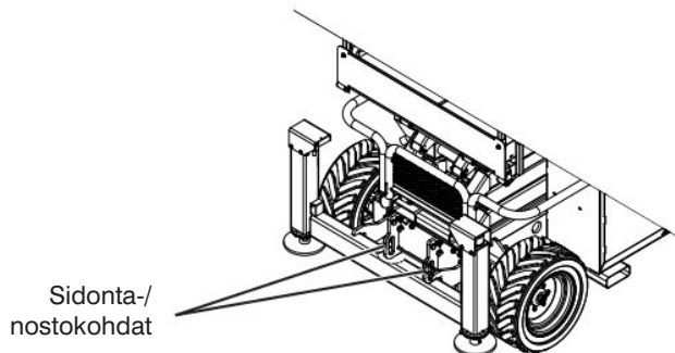
Kuva 3-6. Sidonta-/nostokohdat
