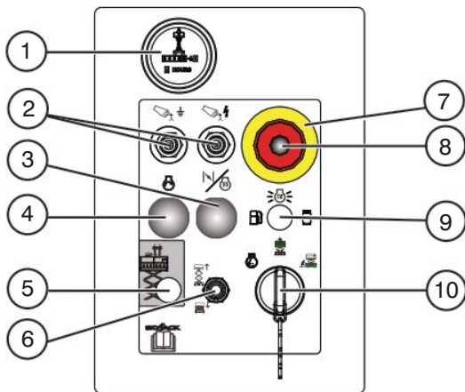
Kuva 2-5. Alustan ohjauspaneeli - Diesel
