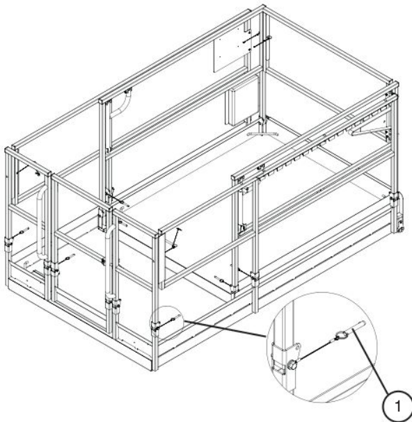
Kuva 3-2. Taitettava suojakaide
