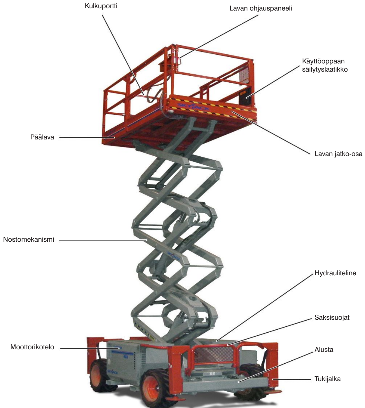
SKYJACK Malli SJ 6832RT Nostolava
