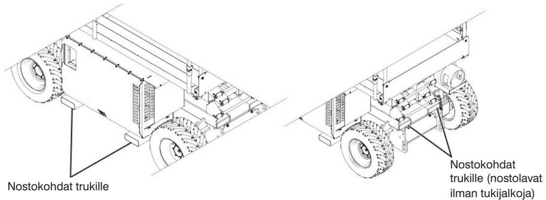
Kuva 3-8. Nostokohdat trukille
