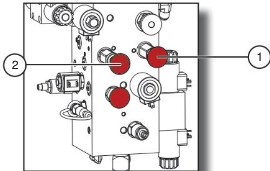
Kuva 2-9. Jarrujärjestelmä
